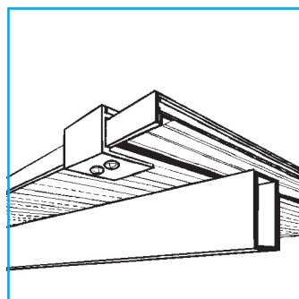
Abb. 8c: Alu-Abschlusswinkel
