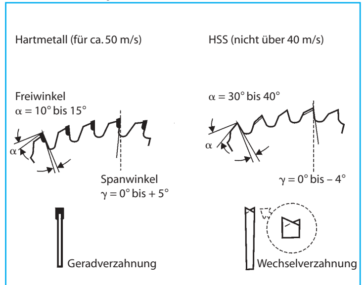
Abb. 6a: Vielzahnsägeblatt
