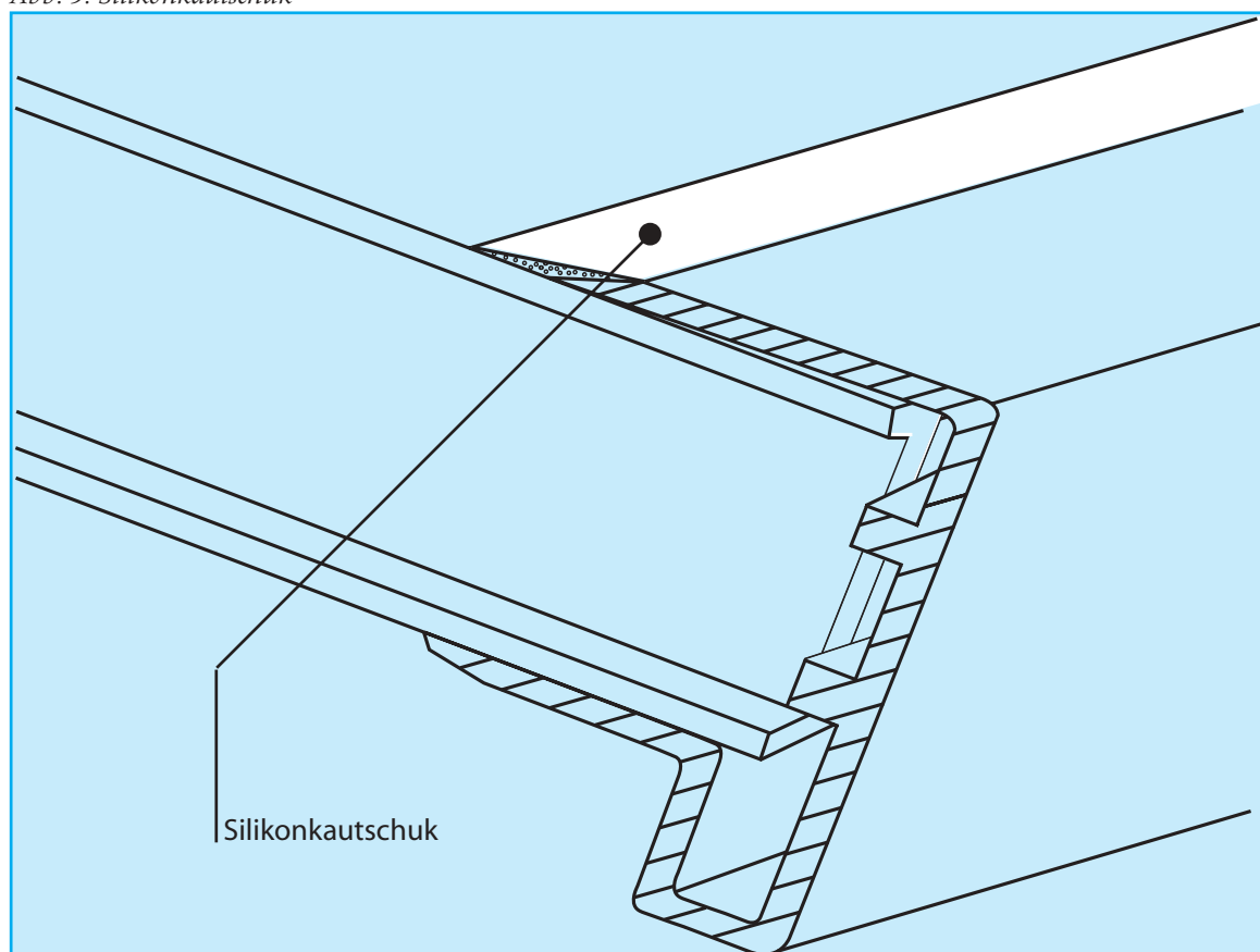
Abb. 5: Silikonkautschuk
