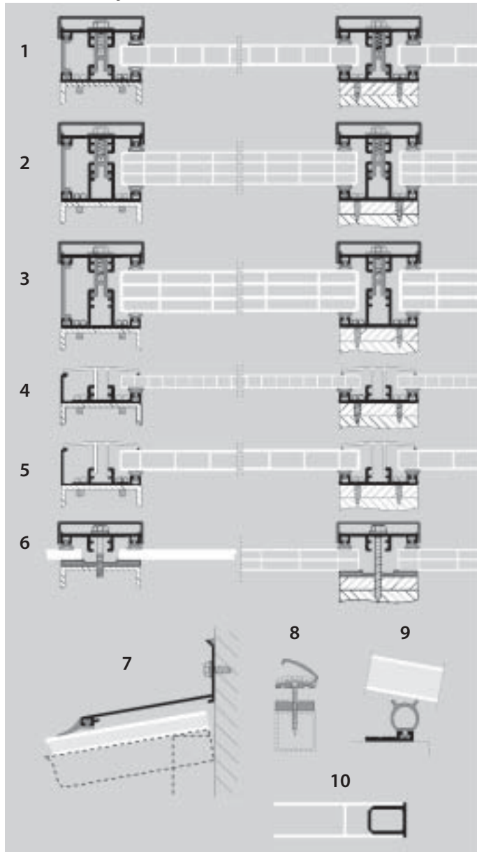
Abb. 8a: Montagezubehör von Röhm
